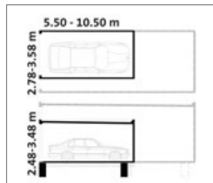
Vue en plan et coupe d'un garage de grandes dimensions
